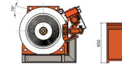
VISTA LATERAL
