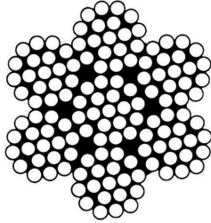
3/16" X 1', 7x19, Galvanized Cable Reel Item #:21015100
